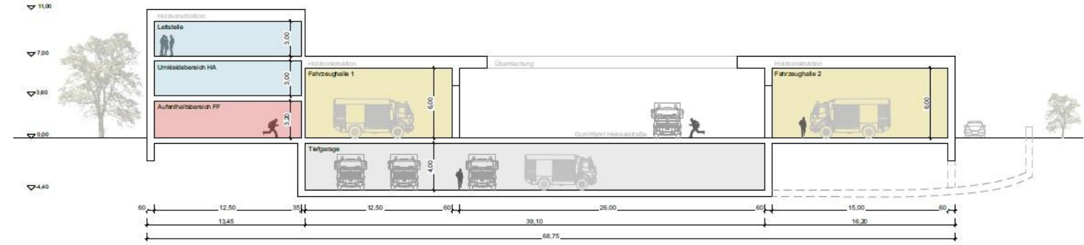
Schnitt A-A M 1:250
