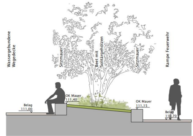
Schnitt C-C'
