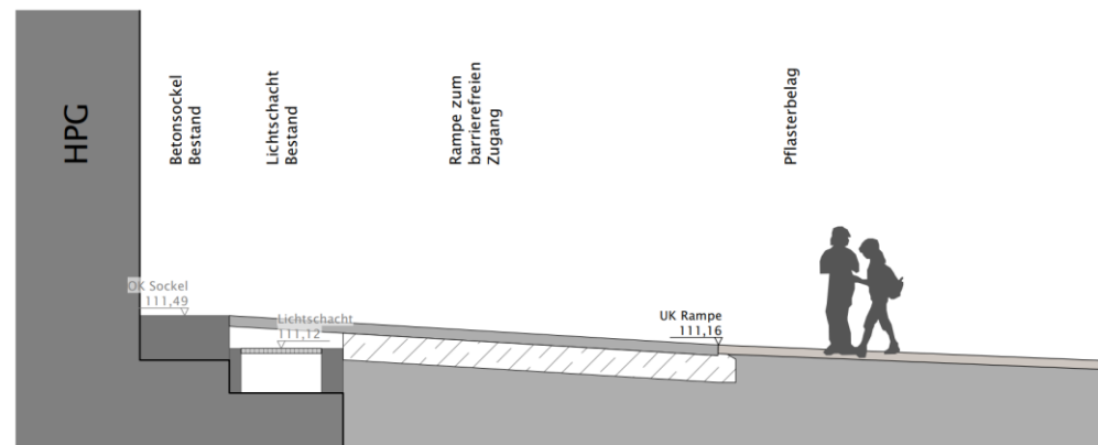
Schnitt I-I'
