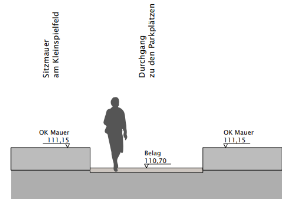
Schnitt G-G'
