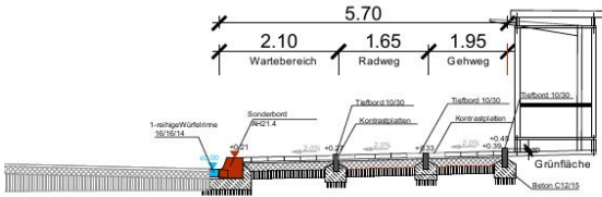
Systemschnitt A-A 1:50
