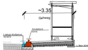
Systemschnitt B-B 1:50
