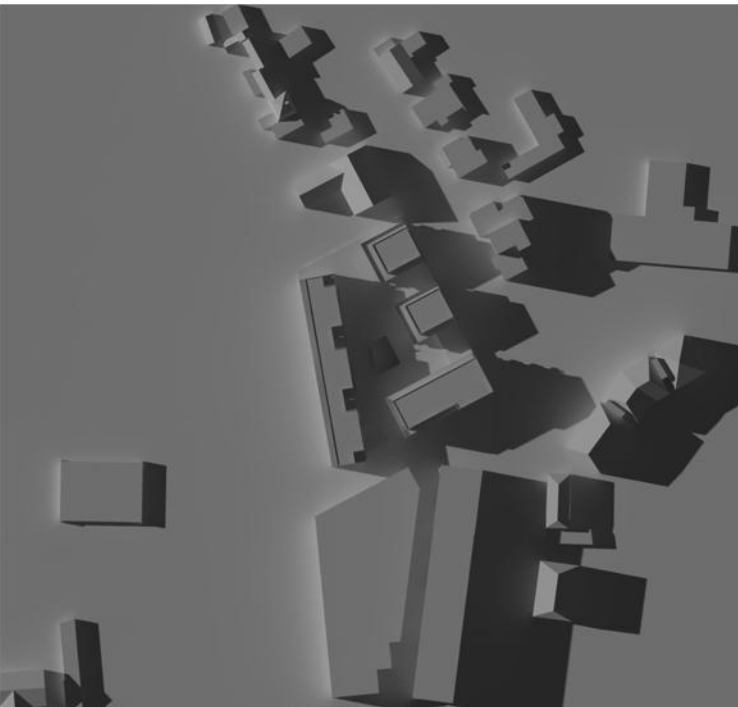
18 Uhr Dämmerung, fast keine Verschattung der Nachbarbebauung gegeben Schatten fällt auf die Straße
