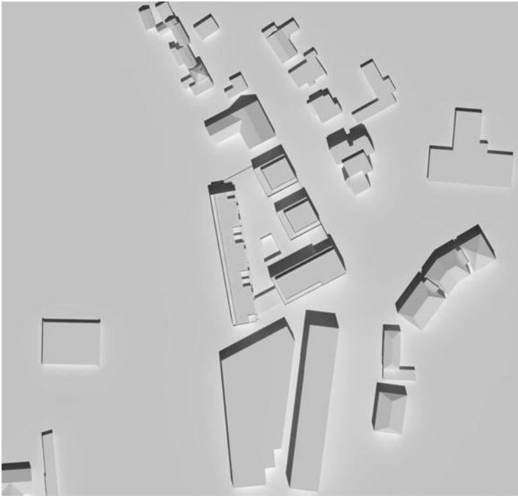
12 Uhr Sonne steht im Süden, keine Verschattung der Nachbarbebauung gegeben
