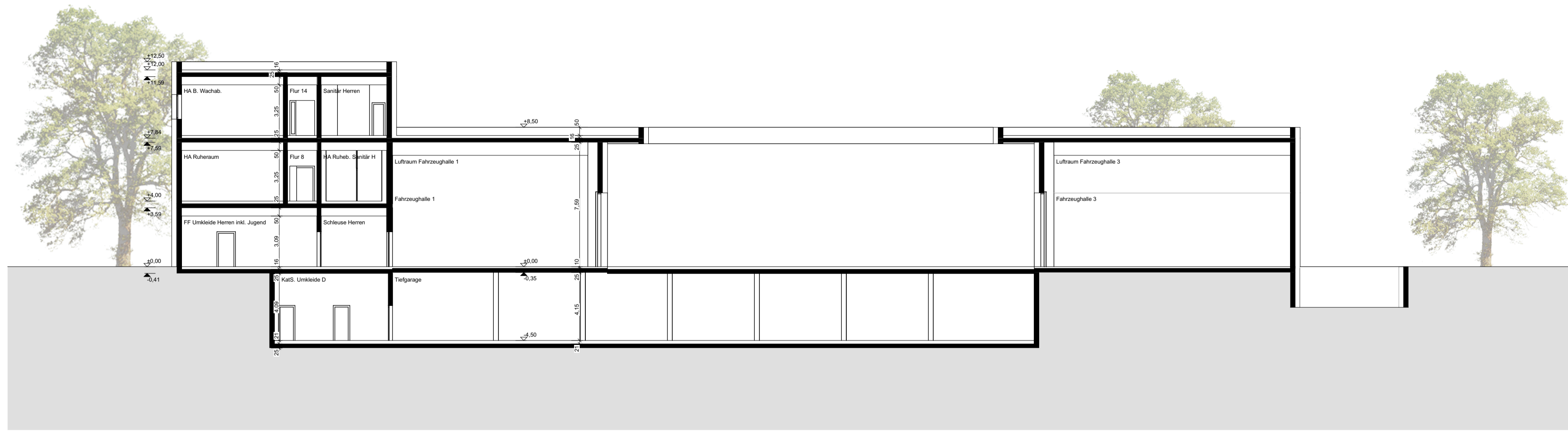
Schnitt A-A
