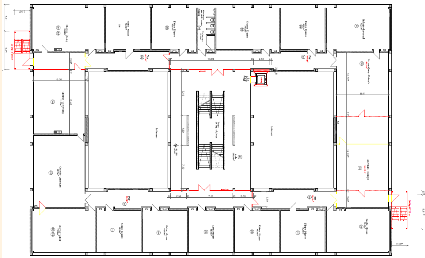
Schematische Darstellung - Brandschutzmaßname HPG
