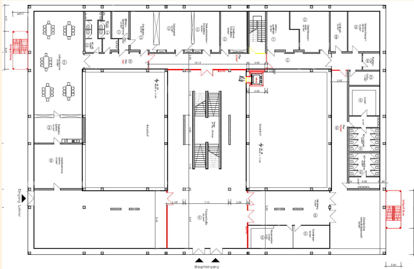
Schematische Darstellung - Brandschutzmaßname HPG
