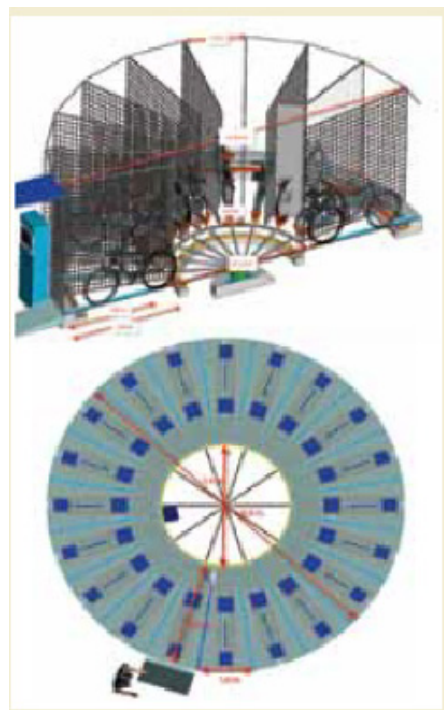
technischer Aufbau und Anordnung Innenraum
